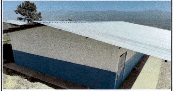
Cubierta de lámina troquelada aluzinc calibre 26 de la nueva bodega escolar.
